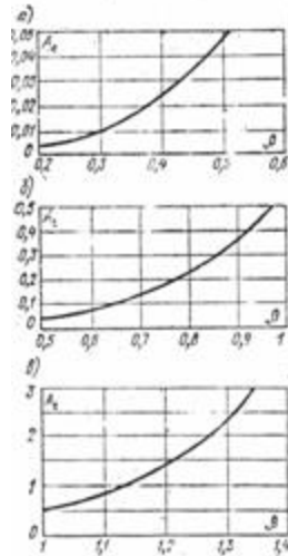
Рис. 2. Зависимость коэффициента b от параметра A_t
