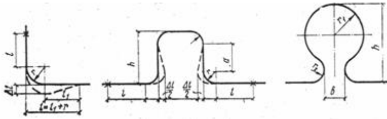
Рис. 3. Основные геометрические параметры
