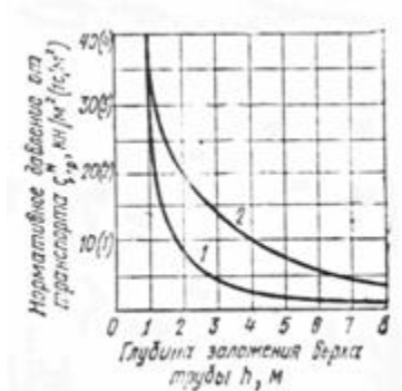
Рис. 1 Зависимость нормативного равномерно распределенного давления транспорта q_{тр}^H от глубины заложения трубопровода
